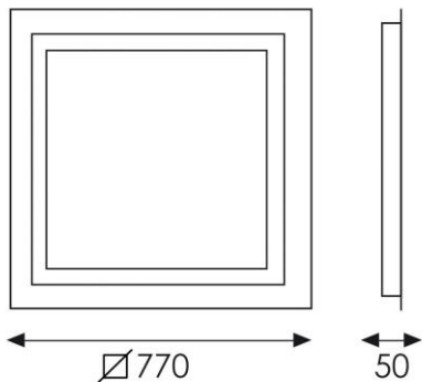
IL 102006 Mirror Light 4xT8 18W IP44
